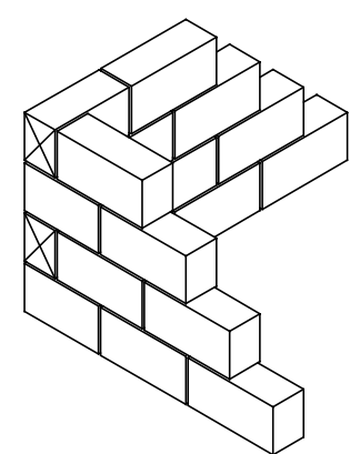
DETALHE DE AMARRAÇÃO EM "L"
