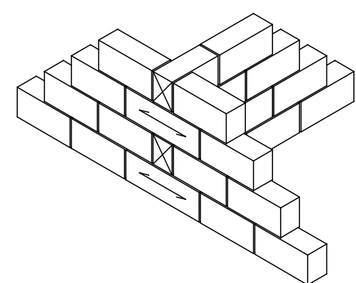
DETALHE DE AMARRAÇÃO EM "T"
